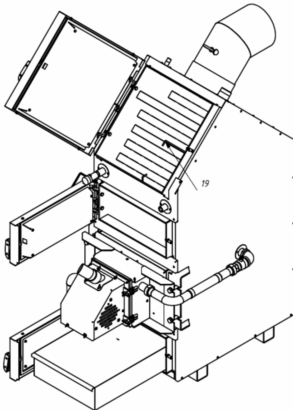
Рис.3. Последовательность операций при очистке котла от золы.
