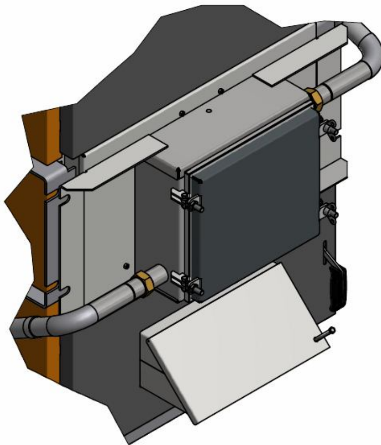
Рис. 7 Установка заглушки для работы на дровах
